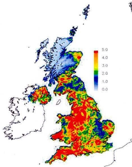
Fig. 3.3(d) FRAME 2002 \text{NH}_x dry deposition [ \text{kg N ha}^{-1} \text{yr}^{-1} ]
