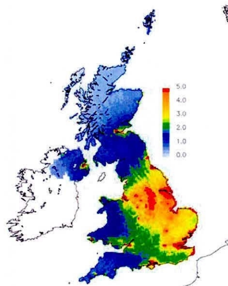
Fig. 3.1(d) FRAME 2002 SO x dry deposition [kg S ha -1 yr -1 ]
