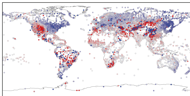
(d) 20CRv3, 1980
